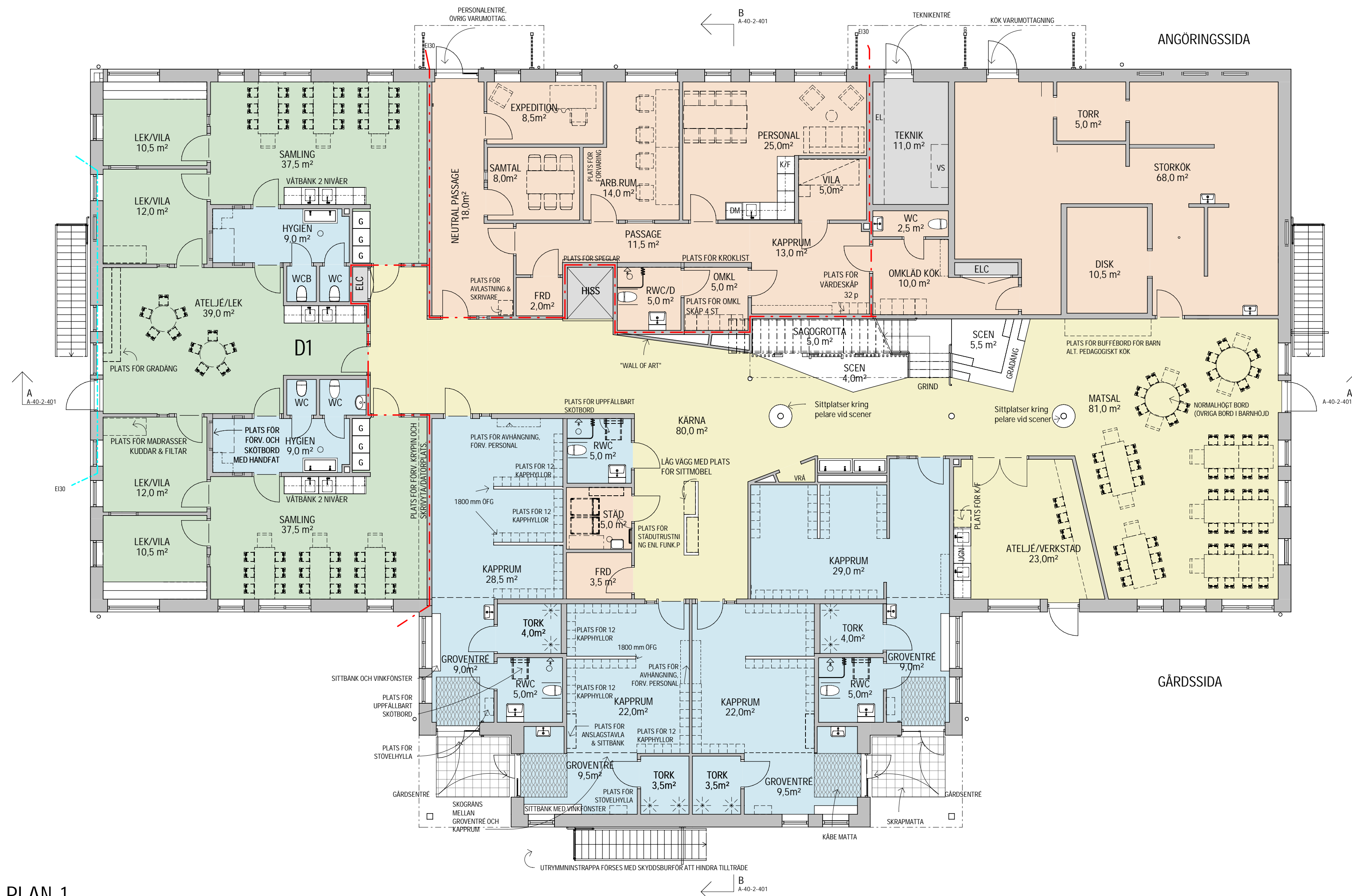
PLAN 1 1 : 100
